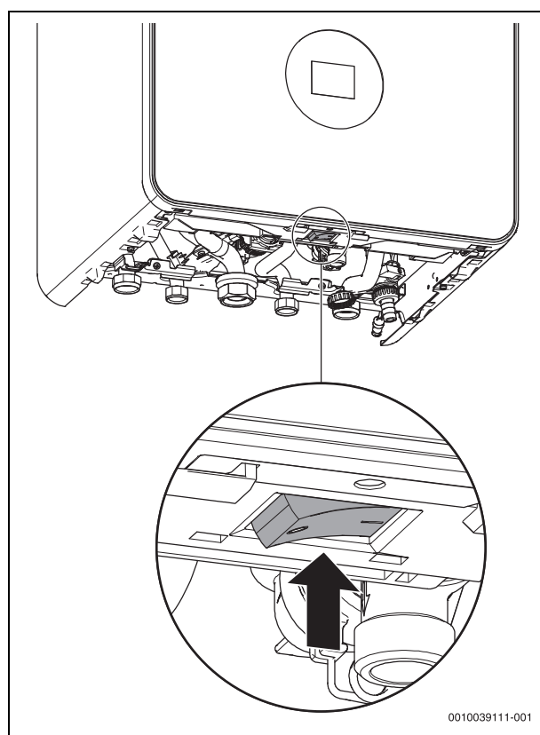
Afb. 1 Aan-uitschakelaar
