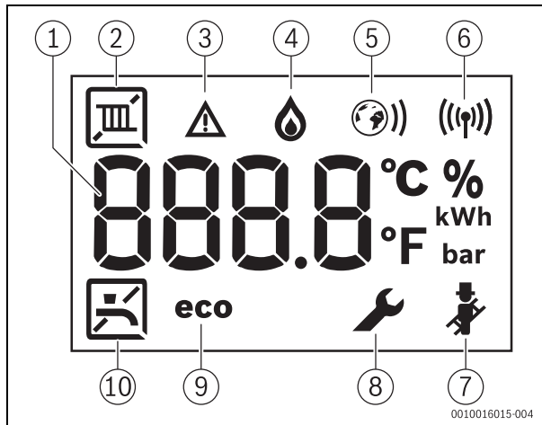
Afb. 3 Displaymeldingen
