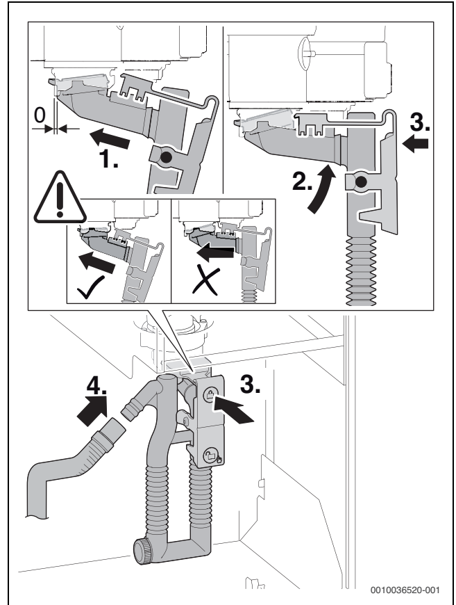
Afb. 66 Condenssifon plaatsen
