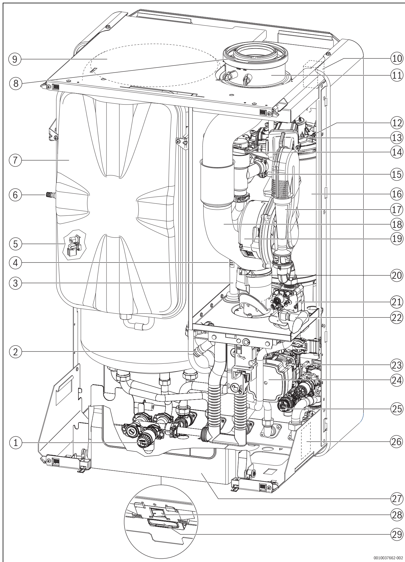
Afb. 4 Productoverzicht
