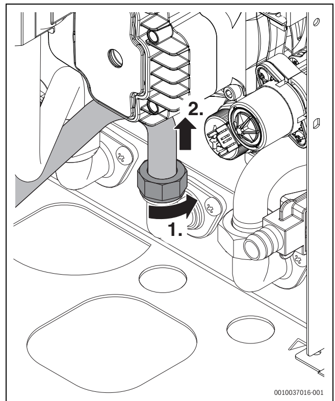
Afb. 67 Buis op koudwateraansluiting afnemen
