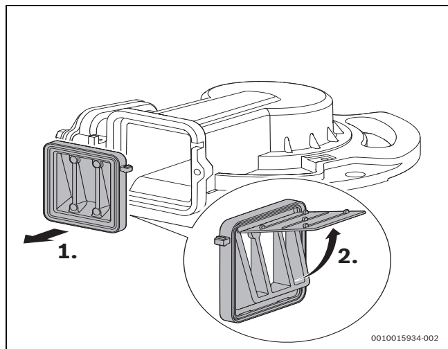
Afb. 52 Terugslagklep in de menginrichting
