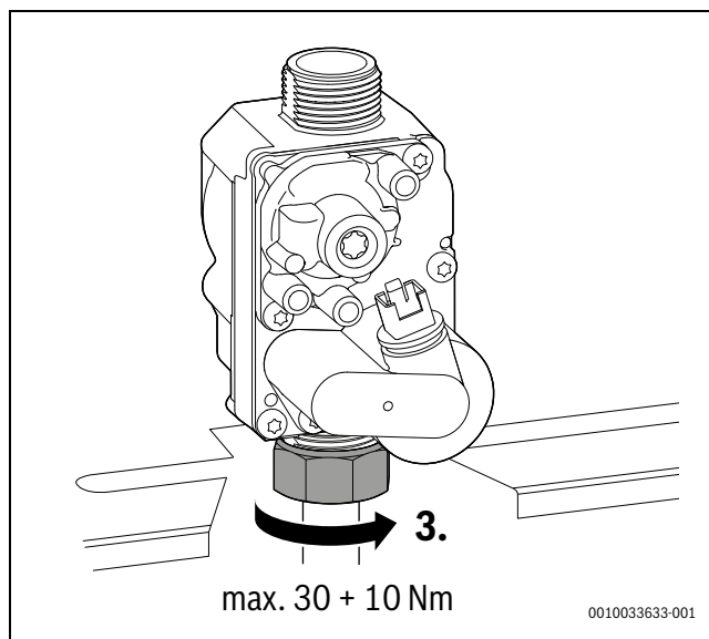
Afb. 74 Draaimoment aanhouden
