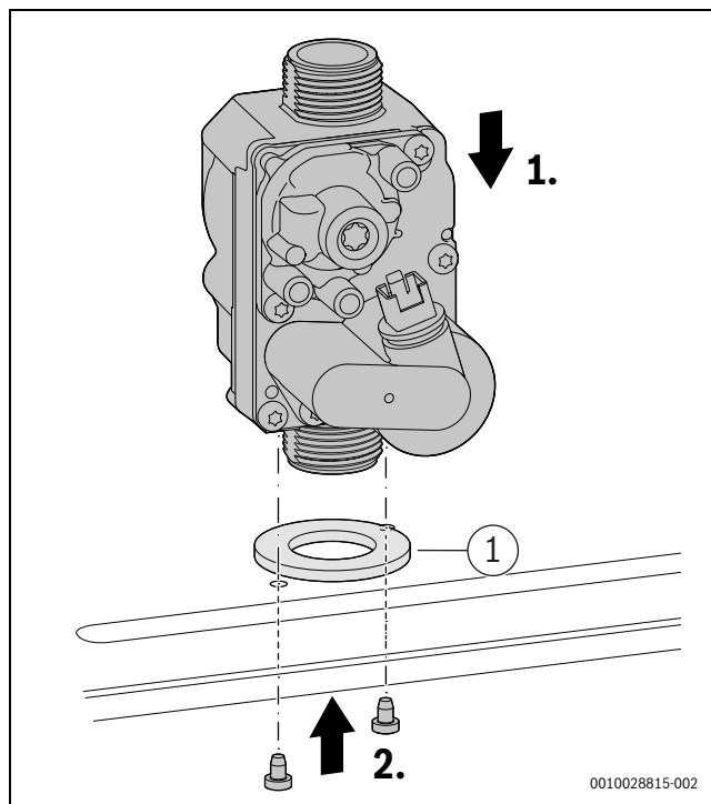
Afb. 73 Gasblok inbouwen
