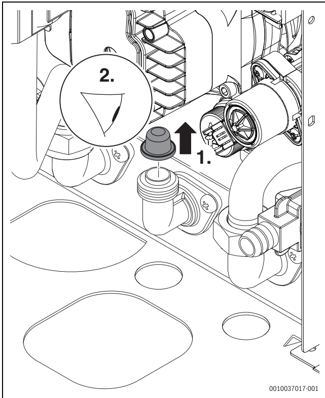
Afb. 68 Controleren filter in koudwaterleiding
