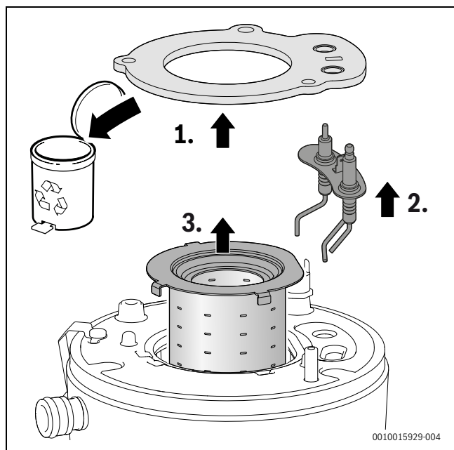
Afb. 53 Brander wegnemen
