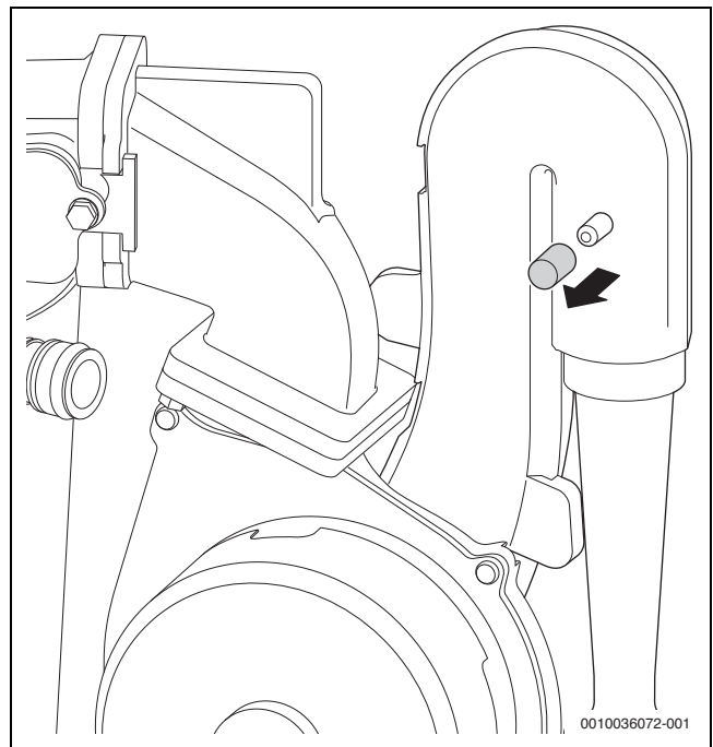
Afb. 48 Meetnippel op de menginrichting
