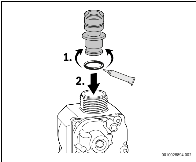
Afb. 75 Gassmoorklep plaatsen
