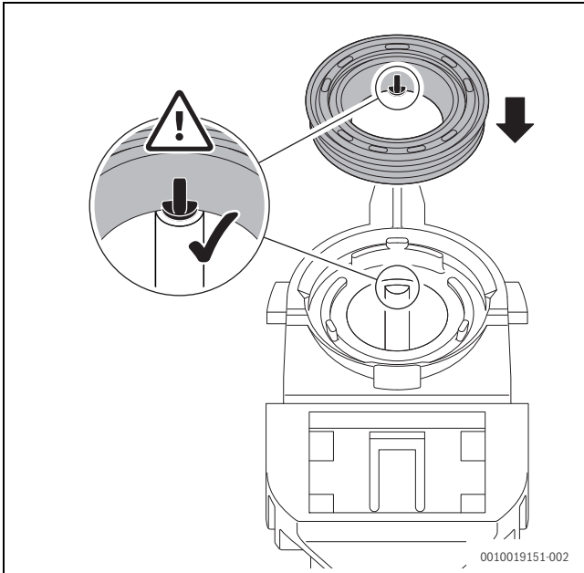
Afb. 64 Dichting correct op de condenssifon plaatsen
