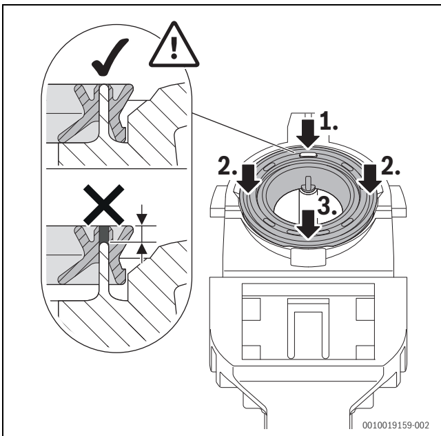
Afb. 65 Dichting aandrukken
