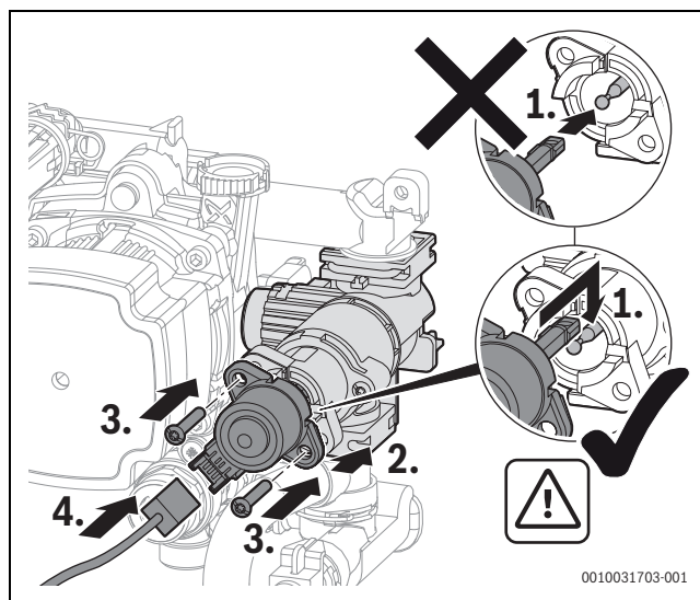
Afb. 80 Motor van de 3-wegklep inbouwen (variant met schroeven)
