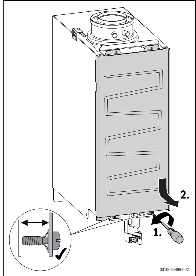
Afb. 44 Branderkap verwijderen
