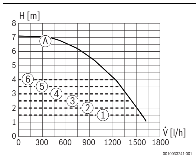
Afb. 81 Pompkarakteristieken en pompcurven
