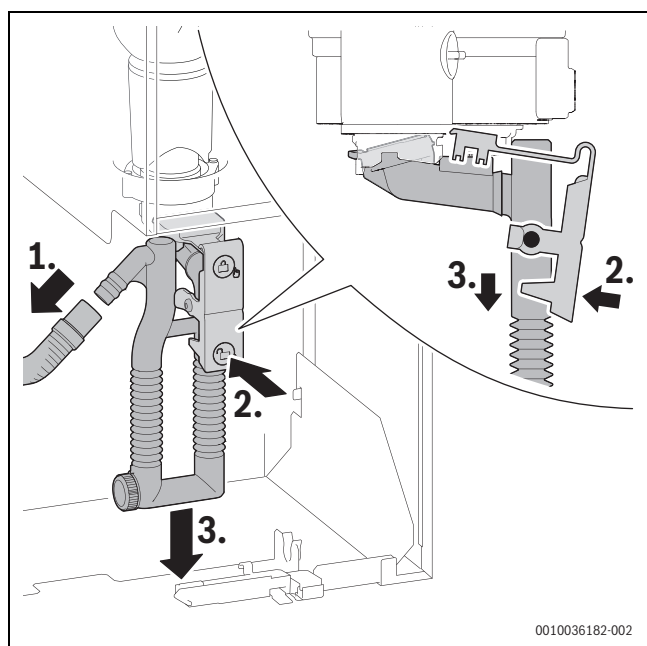
Afb. 61 Condenssifon demonteren
