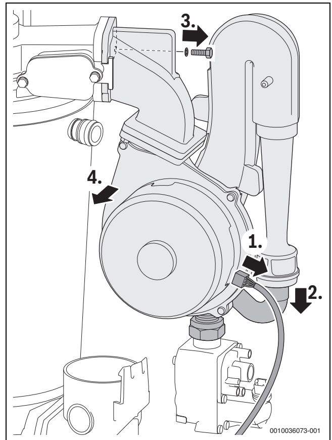
Afb. 50 Ventilator met menginrichting demonteren
