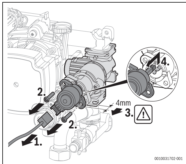
Afb. 79 Motor van de 3-wegklep uitbouwen (variant met schroeven)
