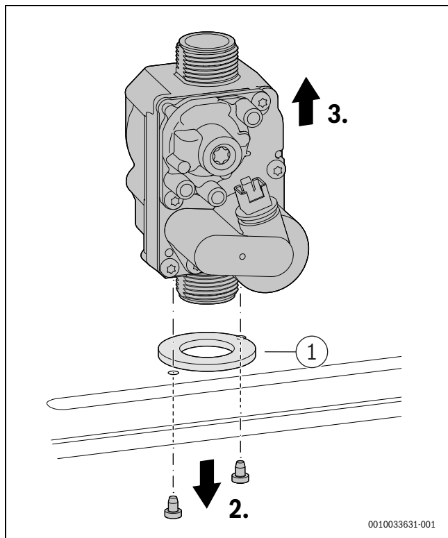
Afb. 72 Gasblok demonteren
