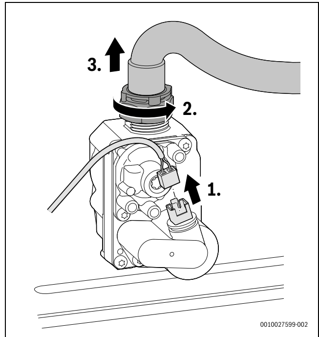
Afb. 69 Stekker op het gasblok lostrekken en wartelmoer met gasslang afnemen
