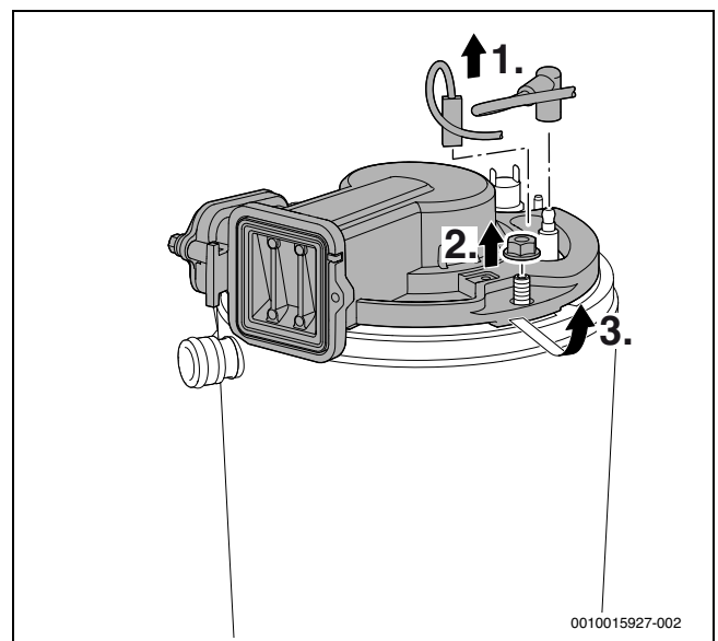
Afb. 51 Branderdeksel losmaken
