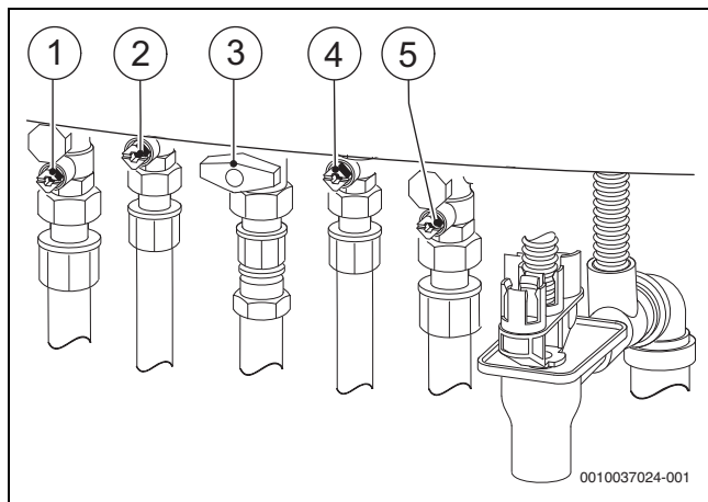
Afb. 38 Gas- en waterzijdige aansluitingen
