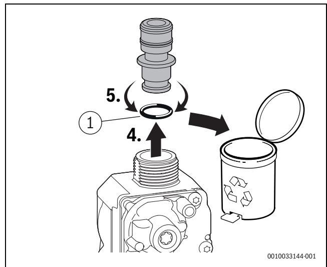
Afb. 70 Gassmoorklep afnemen
