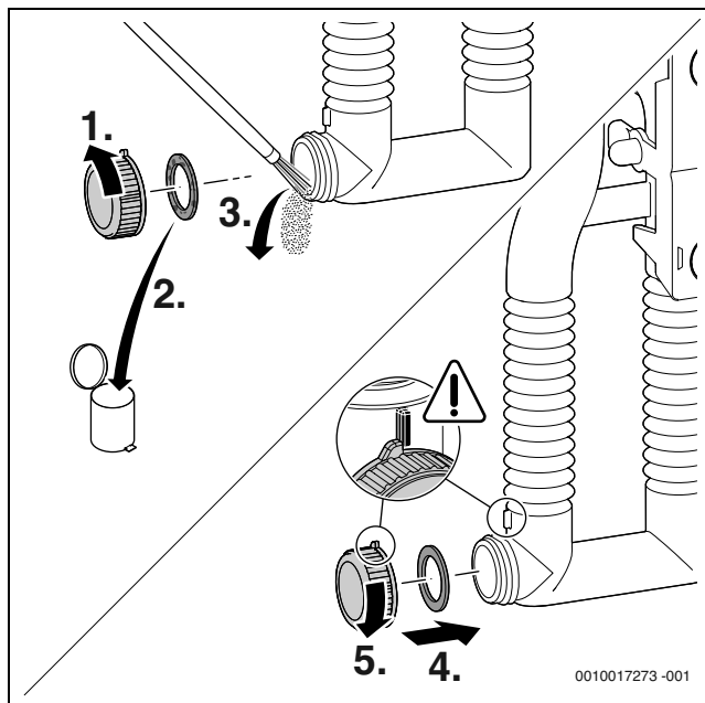
Afb. 62 Condenssifon reinigen
