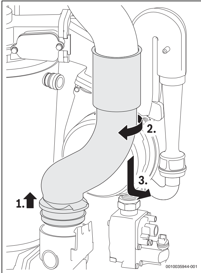
Afb. 49 Rookgasafvoerbuis demonteren
